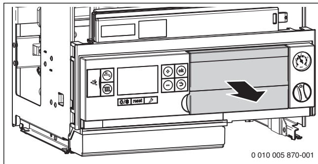
Рис. 29 Удаление крышки и установка пульта управления
