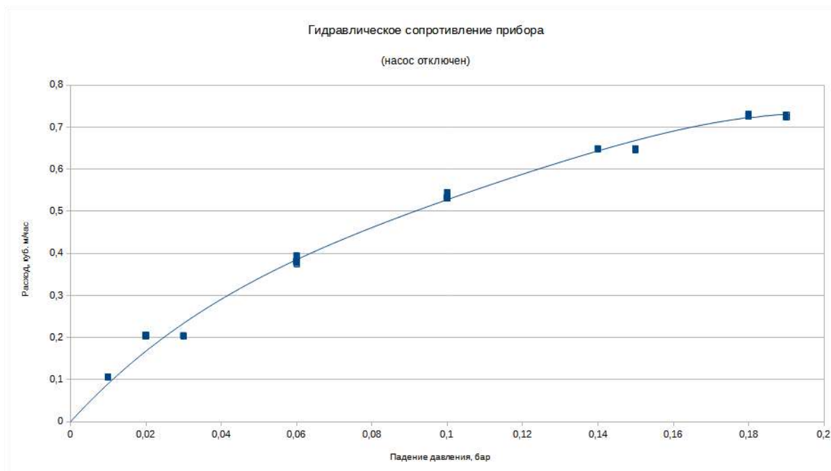
Рисунок 22. Гидравлическое сопротивление прибора
