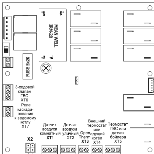
Рисунок 8. Основные разъемы платы управления
